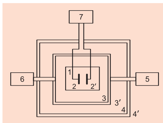
Рис. 3.9 Экспериментальная установка. 1 – кювета с раствором, 2 – электроды, 3 – катушка, 4 – магнитный экран пермаллоя, 5 – источник напряжения, 6 – генератор синусных волн, 7 – измерительный блок: стабилизатор напряжения, измеритель, записывающее устройство [22]
