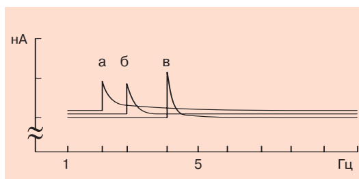
Рис. 3.10 Поток ионов в растворе глутаминовой кислоты как функция частоты переменного магнитного поля для различных значений постоянного магнитного поля. По оси x – частота переменного магнитного поля (Гц), по оси y – поток ионов (нА). Амплитуда переменного магнитного поля равна 0,025 мкТ; постоянное магнитное поле а: V_0 = 20 мкТ; б: V_0 = 30 мкТ; в: V_0 = 40 мкТ
