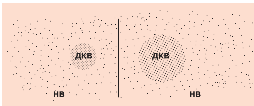
Рис. 3.8. При нагревании, а также под воздействием некоторых физических, химических и фармакологических агентов диаметр доменов когерентности молекул воды существенно уменьшается (слева). При охлаждении и воздействии иных физических факторов и фармакологических средств домены когерентности существенно увеличиваются в размерах (справа). В любом случае диаметр доменов H_2O колеблется в диапазоне от долей микрона до 1,5 мкм
