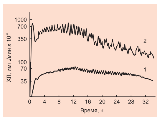
Рис. 3.1. Нелинейная кинетика развития хемилюминесценции (ХЛ) в различных реакционных системах: 1 – (глюкоза–глицин (60 мМ, 60 мМ; 20 мл; pH 11,0); 2 – метилгликоксаль–глицин (10 мМ, 30 мМ; 20 мл; pH 10,6), как пример осцилляторной регуляции
