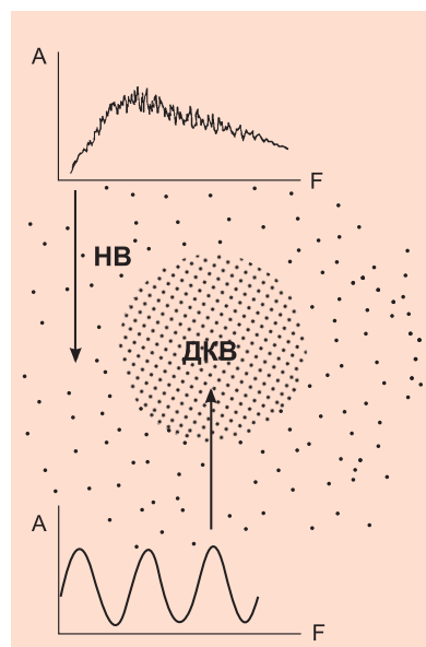
Рис. 3.7. Гипотетическая схема распределения молекул воды в когерентных (ДКВ) и некогерентных (НВ) состояниях. На графиках представлены спектры некогерентных (вверху) состояний и спектр доменов когерентности (внизу) молекул воды
