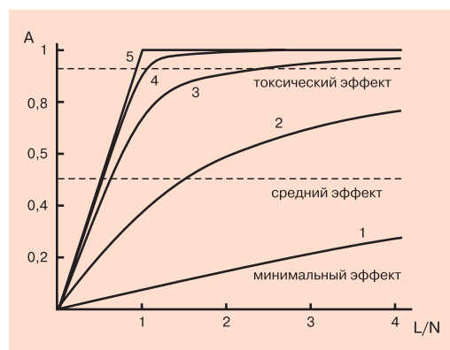
Рис. 3.5. Зависимость активности от мольного соотношения мишеней и молекул лекарств и ксенобиотиков при различных константах равновесия [1]: K_1 = 10^{-8} , K_2 = 10^{-7} , K_3 = 10^{-6} , K_4 = 10^{-5} , K_5 = 1
