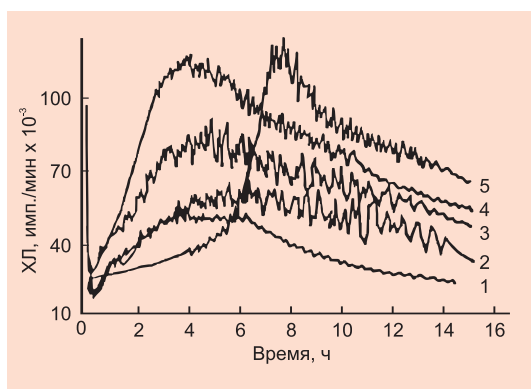
Рис 3.2. Многофазовые регуляторные процессы. Влияние аскорбиновой кислоты на химилюминесценцию (ХЛ) в системе глюкоза–глицин (60 Мм, 60 Мм; 10 МЛ; РН 11,0): 1 – контроль; 2 – 1,0 МКм аскорбата; 3 – 10 МКм аскорбата; 4 – 100МКм аскорбата; 5 – 1000 МКм аскорбата
