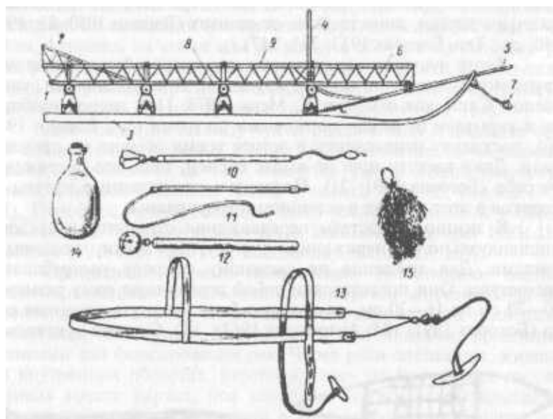
Детали эскимосских нарт, запрягаемых собаками (втор. четв. XX в.):
